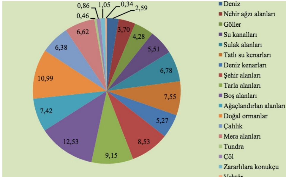
Grafik 1. Dünyadaki İşgalci Yeni Türlerin yaşadıkları habitata göre bulunma oranları(%) (GISD,2015'ten)
